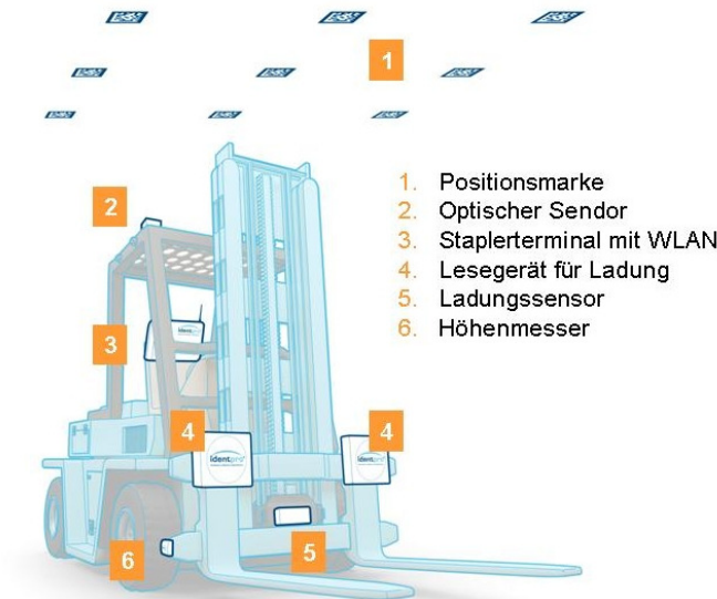
Das identPLUS Lokalisierungssystem von IdentPro mit Option RFID-Ladungserkennung
